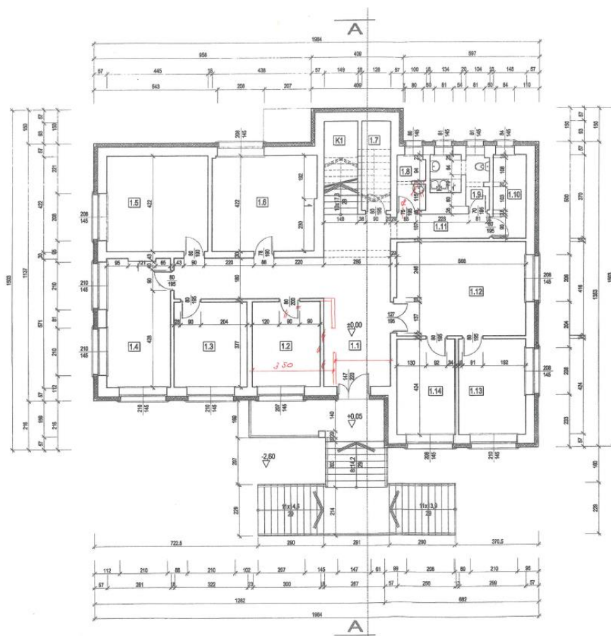
Zdjęcie przedstawia stan projektowany rozkładu pomieszczeń parteru budynku urzędu gminy w Godzieszach Wielkich po wykonaniu prac remontowych
