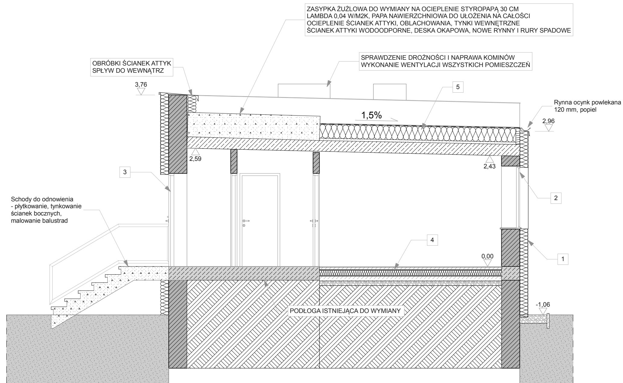
Przekrój 1-1
