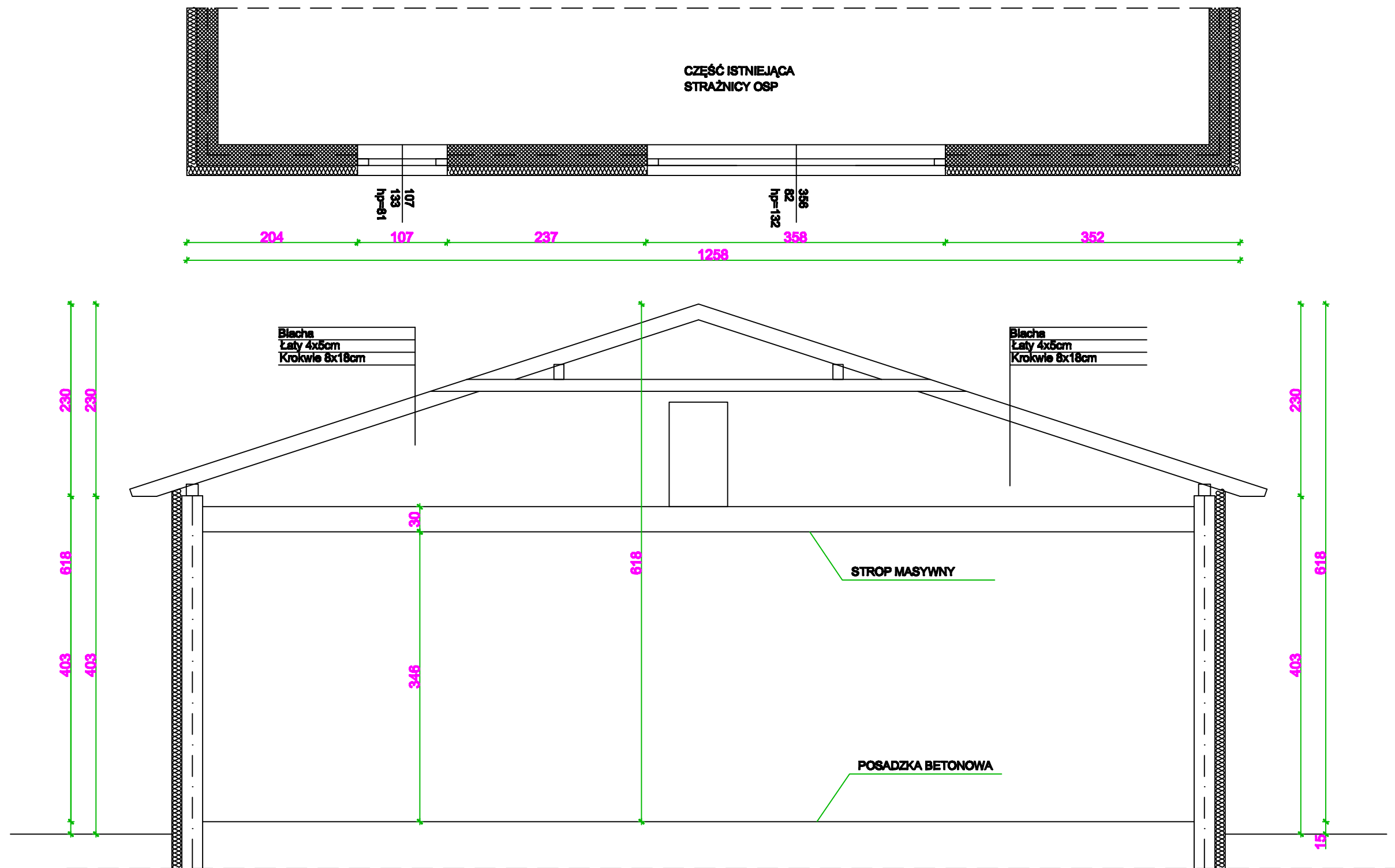
RZUT PRZYZIEMIA I PRZEKRÓJ POPRZECZNY - INWENTARYZACJA - skala 1:50
