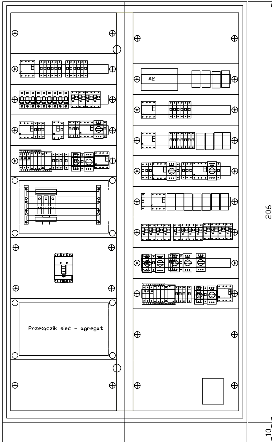
Szafa dwupolowa do zabudowy szeregowej ( 2 x 800 ) typ: XVTL prod. Eaton
